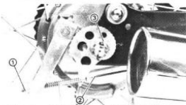
1. Ajustador 2. Varilla del freno 3. Pasador abierto
