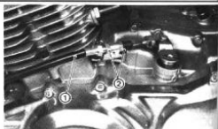
1. Cable del embrague 2. Ajustador / contratuerca
