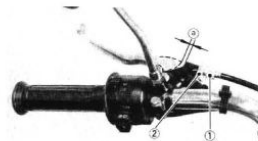
1. Ajustador 2. Contratuerca a. 2 - 3 mm (0.08 - 0.12 pulg)
